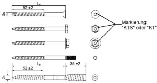
Spezialschraube KT 14
