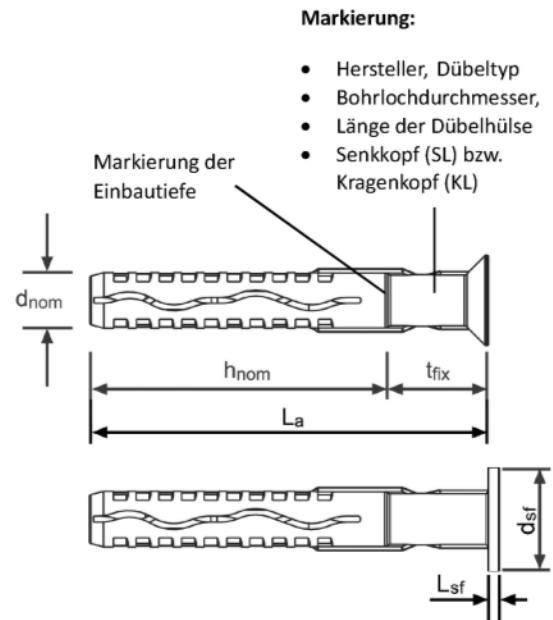
Dübelhülse KT 14
